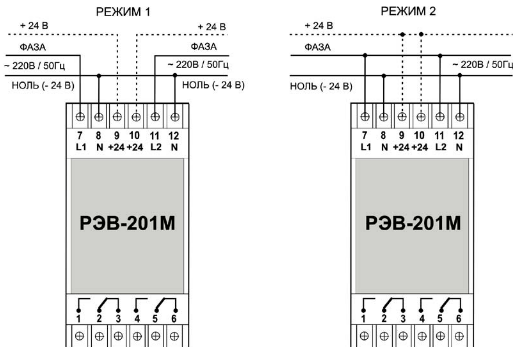
Рисунок 7 – подключение реле в зависимости от режима работы
