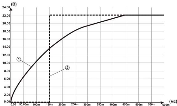
1 – кривая нарастания напряжения источника питания РЭВ-201; 2 – кривая состояния реле нагрузки при нулевых выдержках времени.
