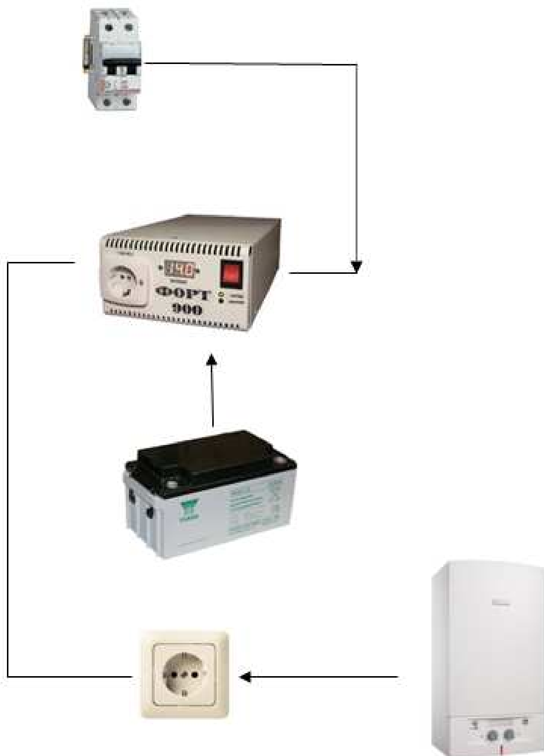
Рис.3. Пример подключения ИБП ФОРТ без использованием стабилизатора
