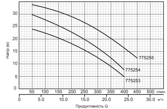
Мал. 2. (продовження) Діаграми продуктивності відцентрових поверхневих насосів.
