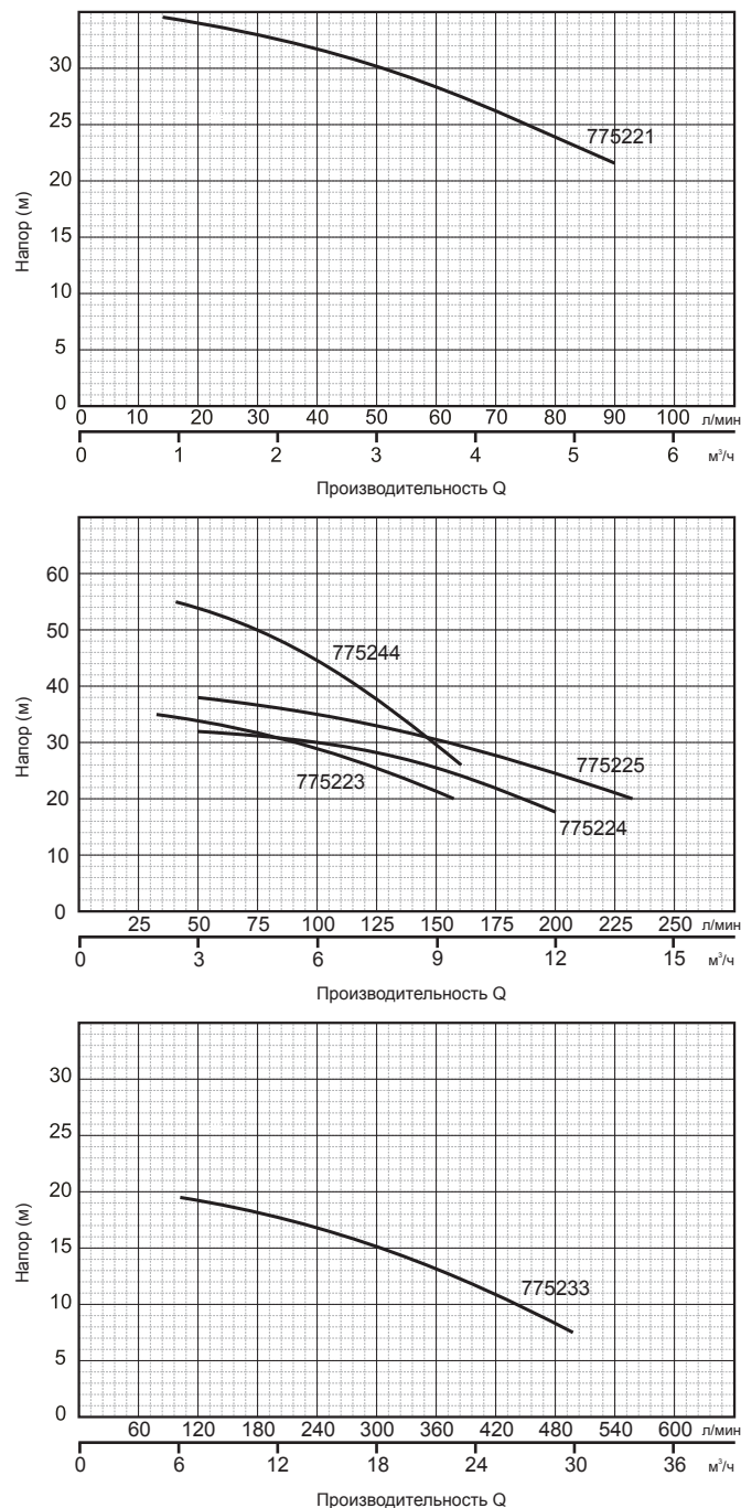
Рис. 2. Диаграммы производительности центробежных поверхностных насосов.
