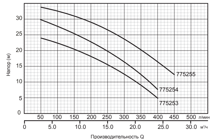
Рис. 2 (продолжение). Диаграммы производительности центробежных поверхностных насосов.
