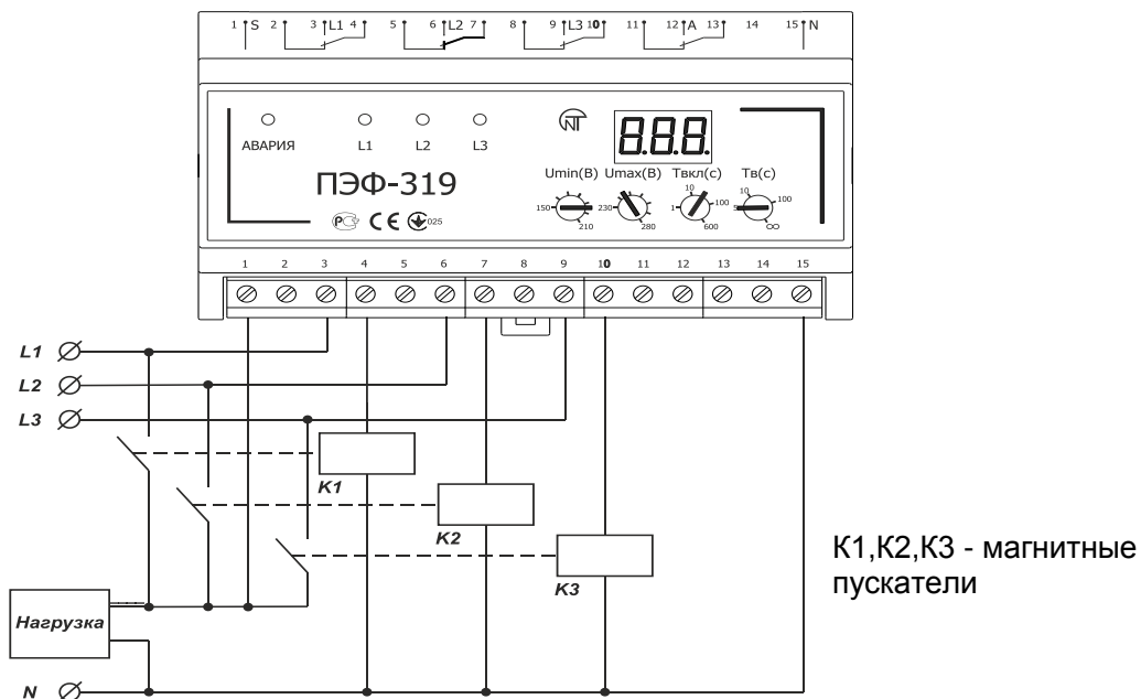
Рисунок 3 – Схема подключения ПЭФ-319 при величине нагрузки более 30 А с использованием магнитных пускателей
