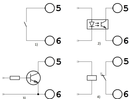
Мал. 3 Варіанти схем зовнішнього керування.
